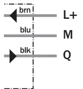
3 x 0.14 mm²
