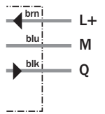
3 x 0.14 mm²
