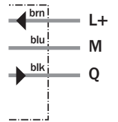
3 x 0.14 mm²
